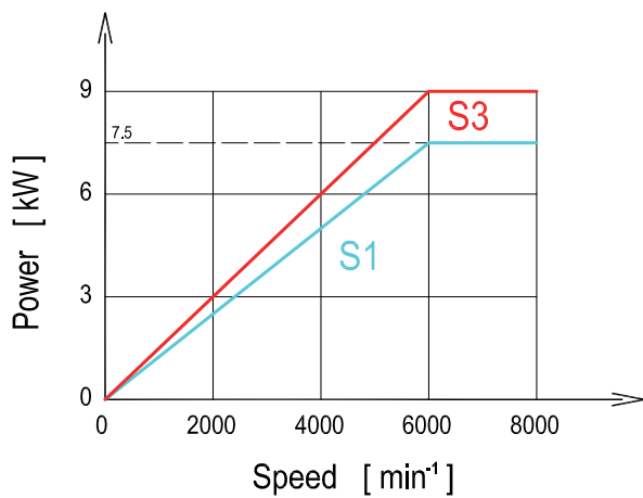
Broche principale à moteur intégré / Hauptspindel mit Integriertmotor / Main spindle with integrated motor
