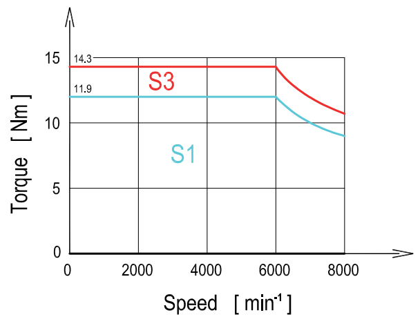
Broche principale à moteur intégré / Hauptspindel mit Integriertmotor / Main spindle with integrated motor
