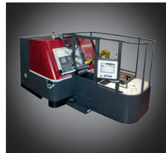
136/142 series Robot Centre de tournage et de production Hochpräzisions-Produktions-Drehcenter High precision and production turning center
